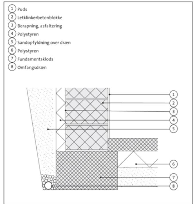
Fig. 410.44. Kælderydervæg af blokke med udvendig isolering.
