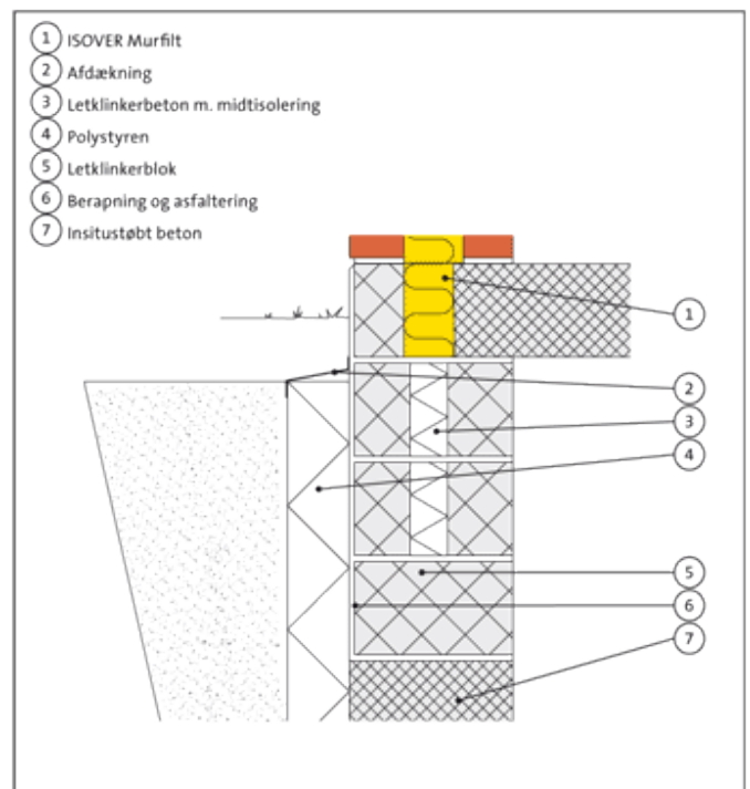
Fig. 410.46. Kælderydervæg/dæk - udvendig isolering.
