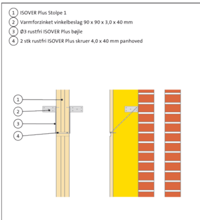
Figur 3. Detalje med U-bøjler.
