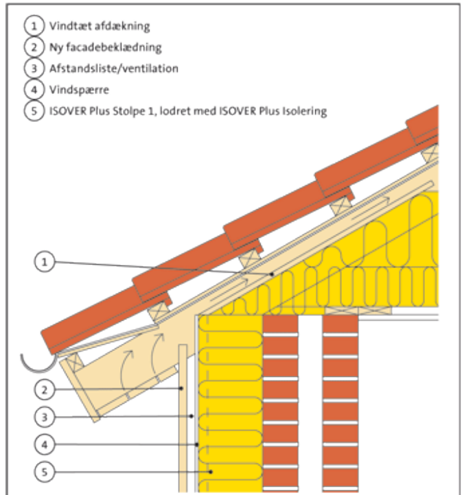
Figur 4. Eksempel på detalje ved udhæng.
