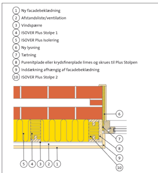
Figur 7. Detalje ved vinduer og døre. Denne placering giver minimalt linietaf.
