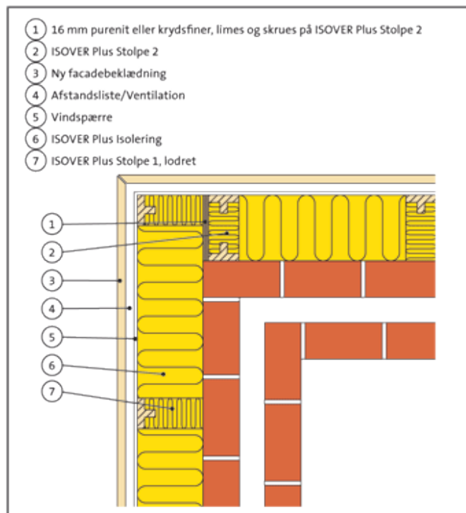
Figur 6. Eksempel på detalje ved udvendig hjørne.
