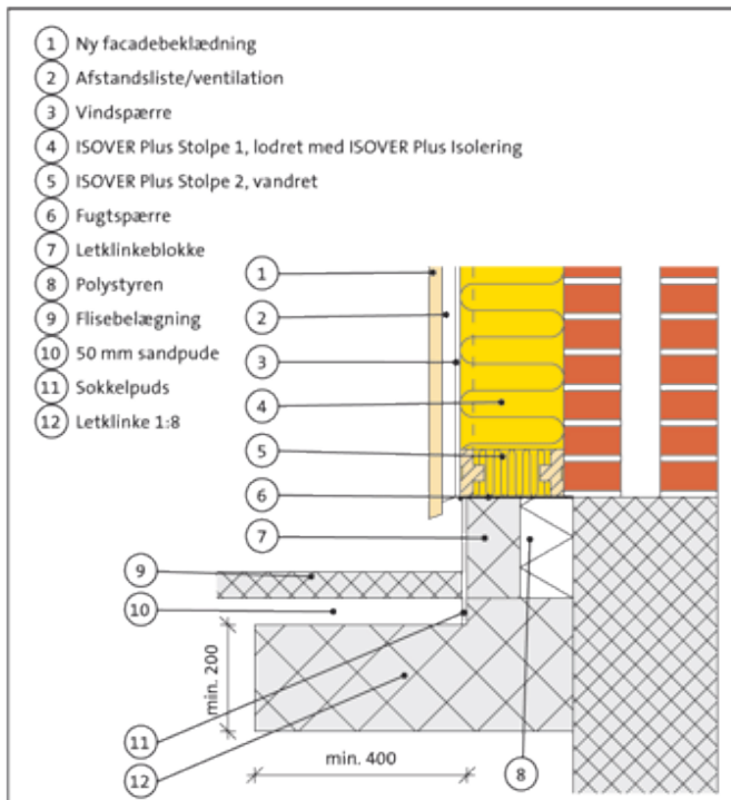
Figur 1. Fundamentsløsning med vandret efterisolering. Denne løsning sikrer at fundamentet ikke hæves ved frostpåvirkning.
