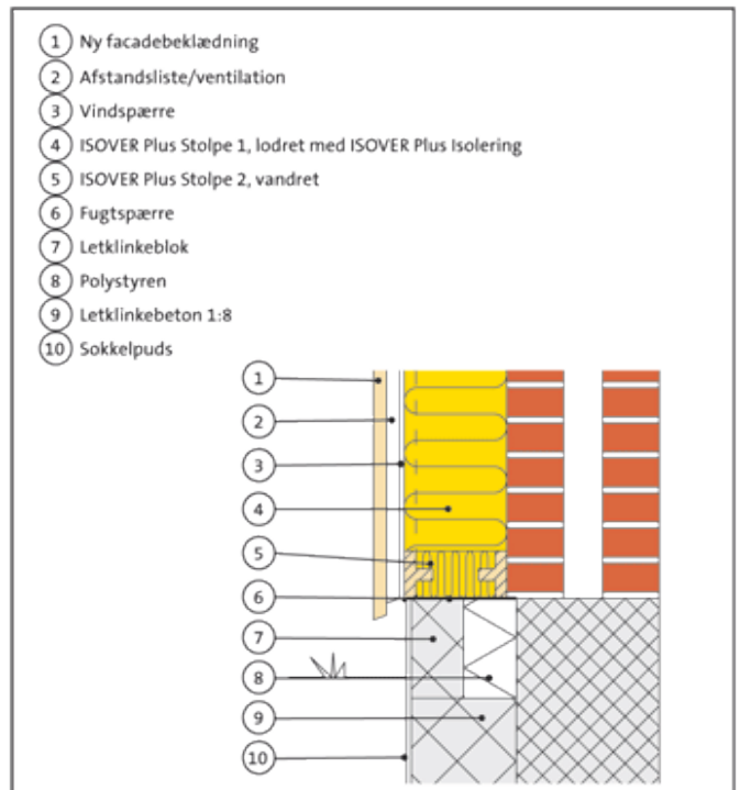
Figur 2. Fundamentsløsning med lodret efterisolering. Denne løsning skal føres til frostfri dybde.
