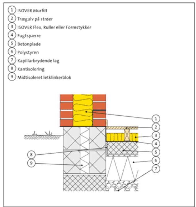
Fig. 410.29. Sokkel/terrændæk - hulmur og trægulv på strøer.
