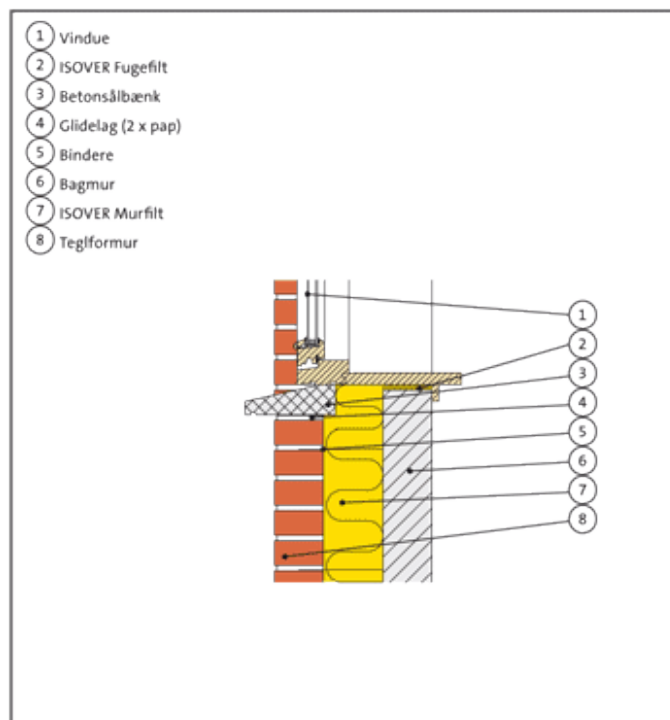
Fig 410.33. Betonsålbænk
