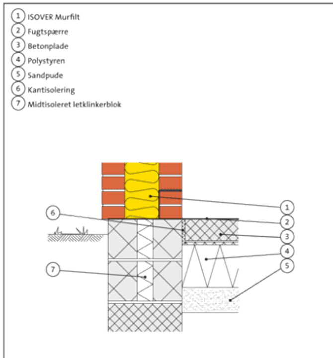
Fig. 410.28. Sokkel/terrændæk - hulmur og klinsegulv el. lign.
