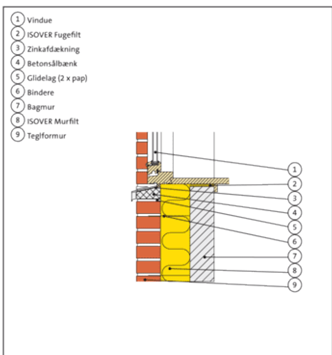
Fig. 410.34. Metalsålbænk.
