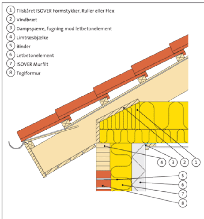
Fig. 410.41. Ydervæg tegl/letbeton.
