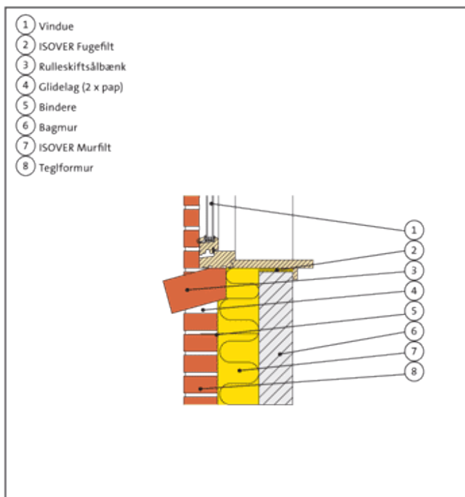
Fig. 410.32. Rulleskiftesålbænk
