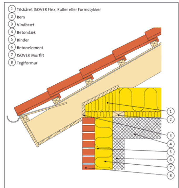
Fig. 410.42. Ydervæg tegl/letbeton med rem.
