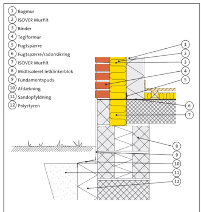
Fig. 410.31. Sokkel/kælderdek - hulmur og trægulv på strøer.
