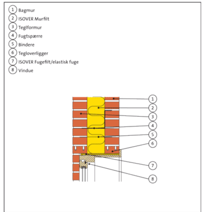
Fig. 410.36. Tegloverligger og lysning i plademateriale.
