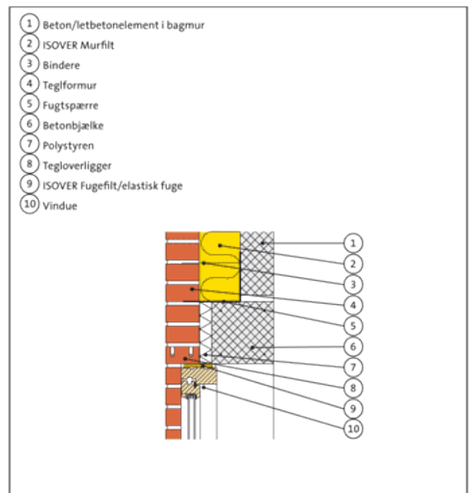
Fig. 410.38. Tegloverligger og bagmur i beton/letbeton og betonbjælke.
