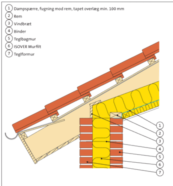
Fig. 410.39. Ydervæg tegl/tegl.
