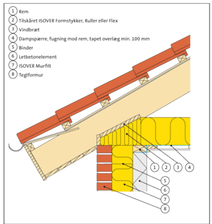
Fig. 410.40. Ydervæg tegl/beton.
